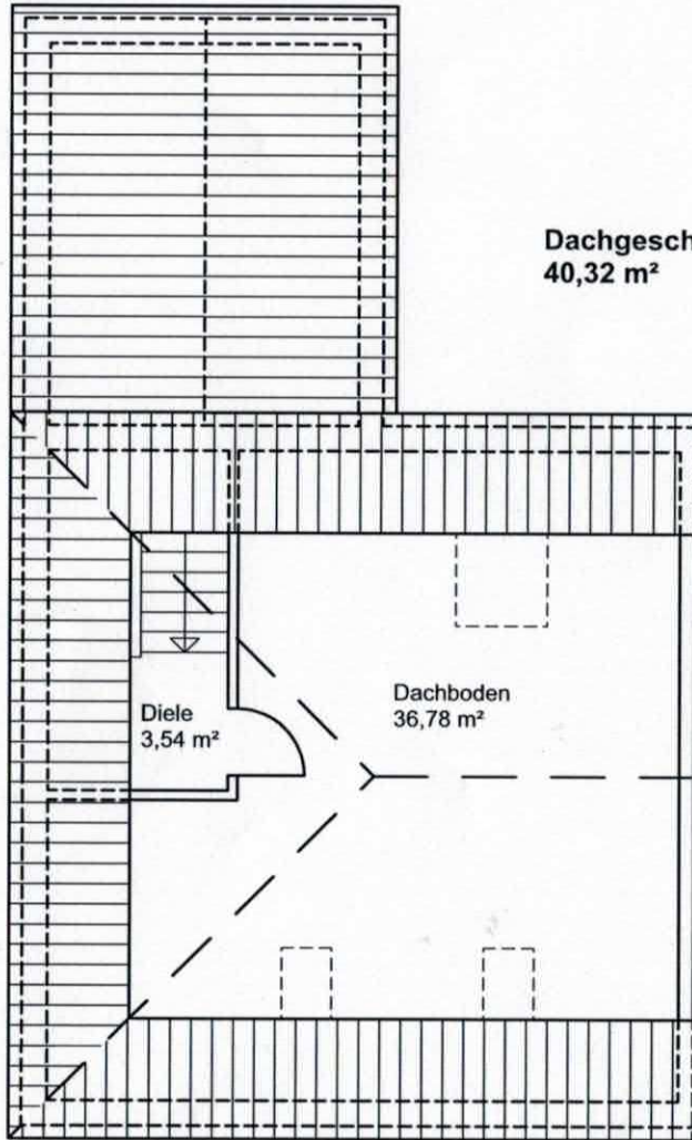
GRUNDRISS DG
