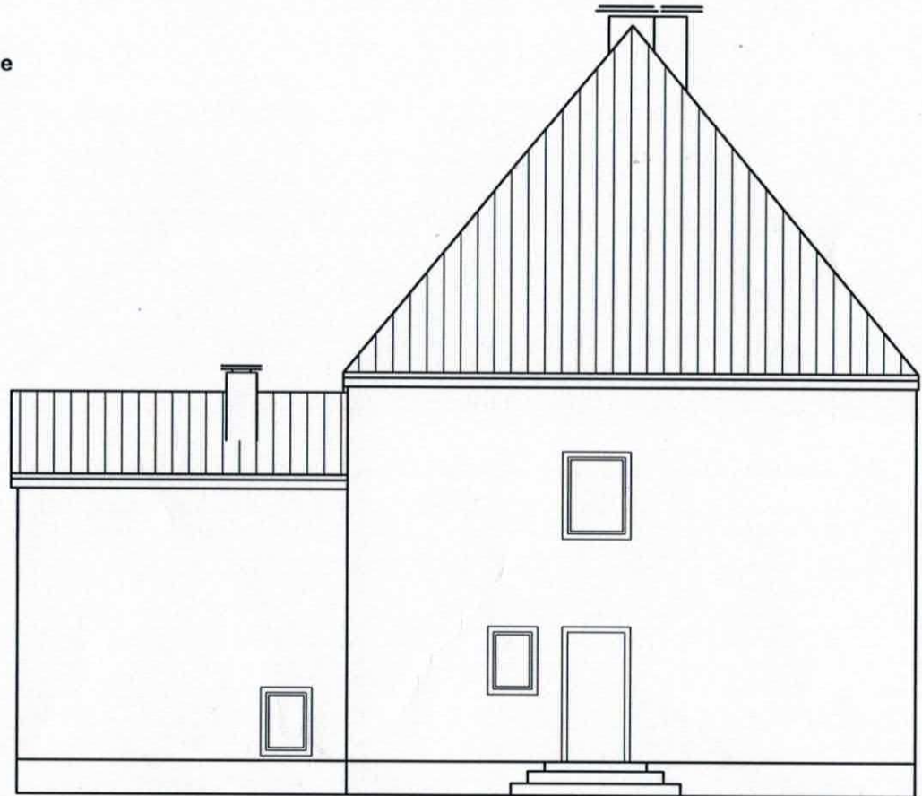
SEITENANSICHT
