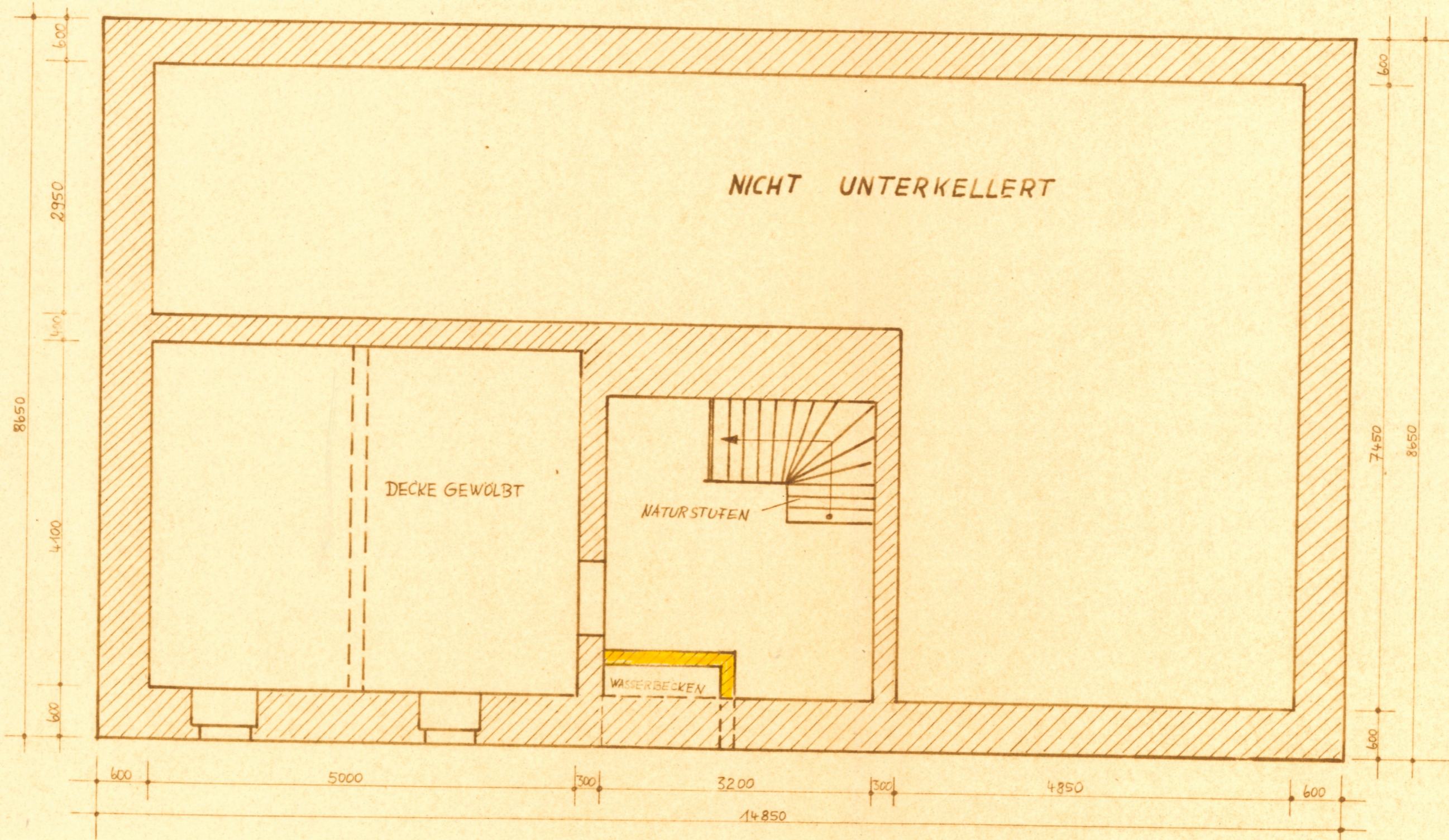
GRUNDRISS KELLER M 1:50
