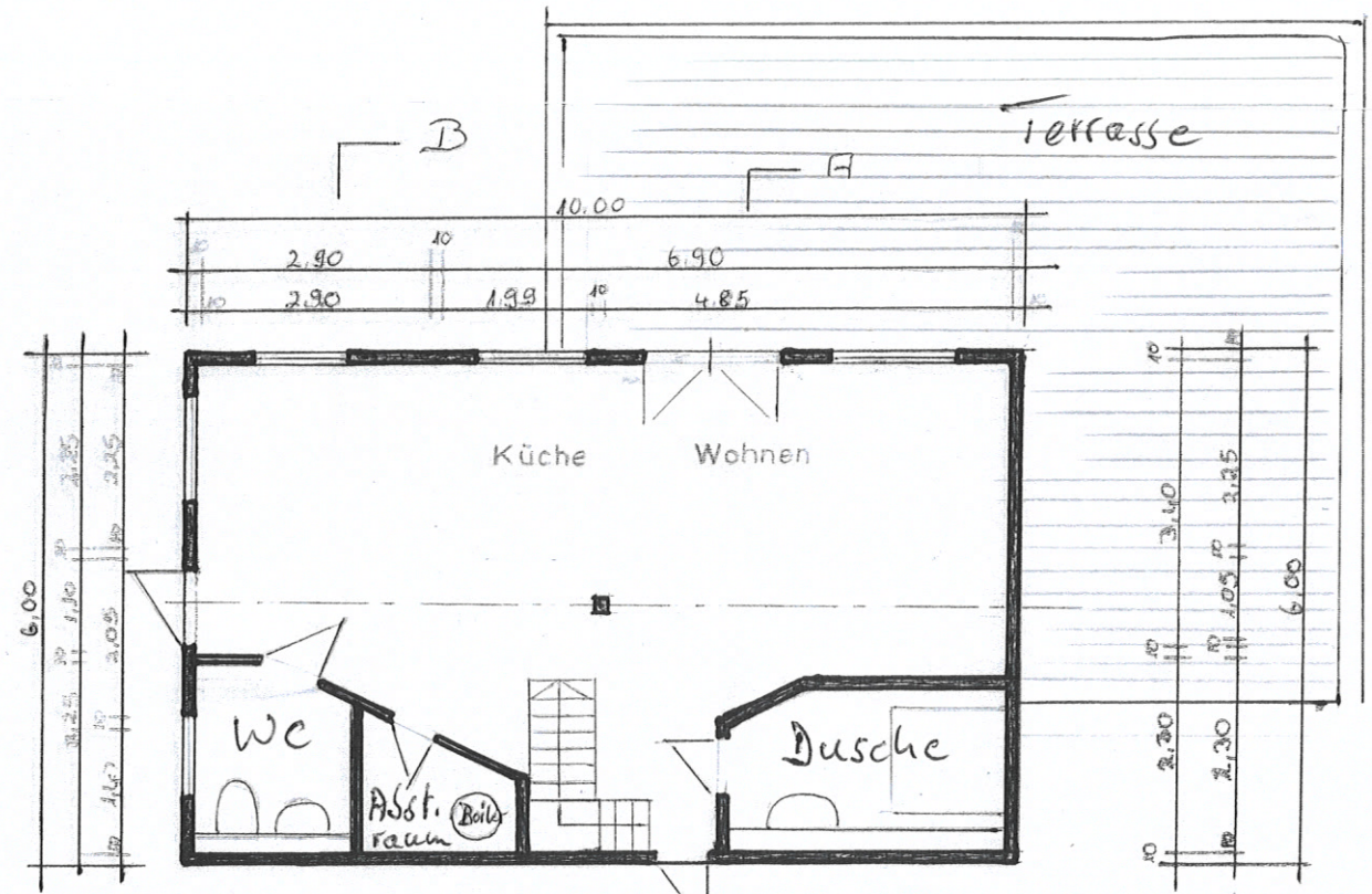
ERDGESCHOSS
