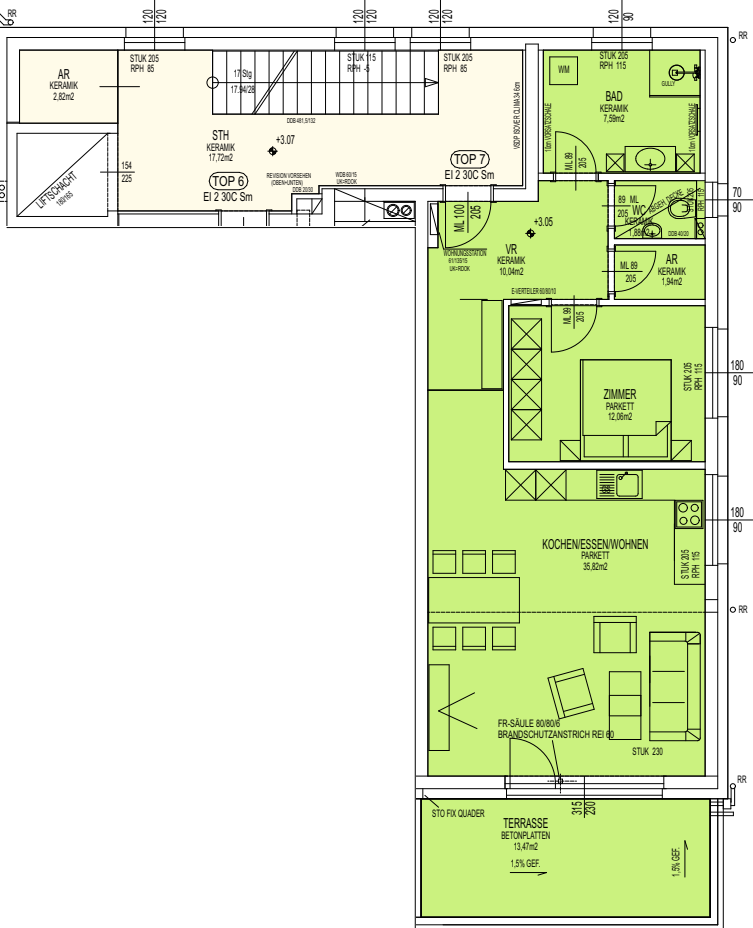
Grundriss 0 1 2 3 4 5m
