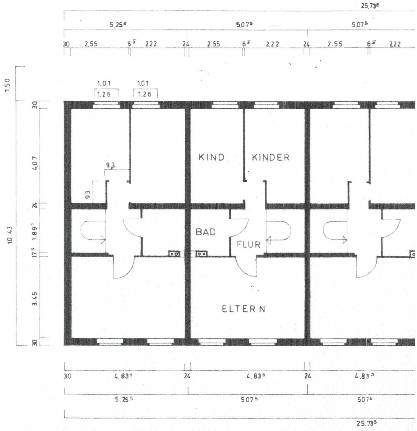
OBERGESCHOSS
