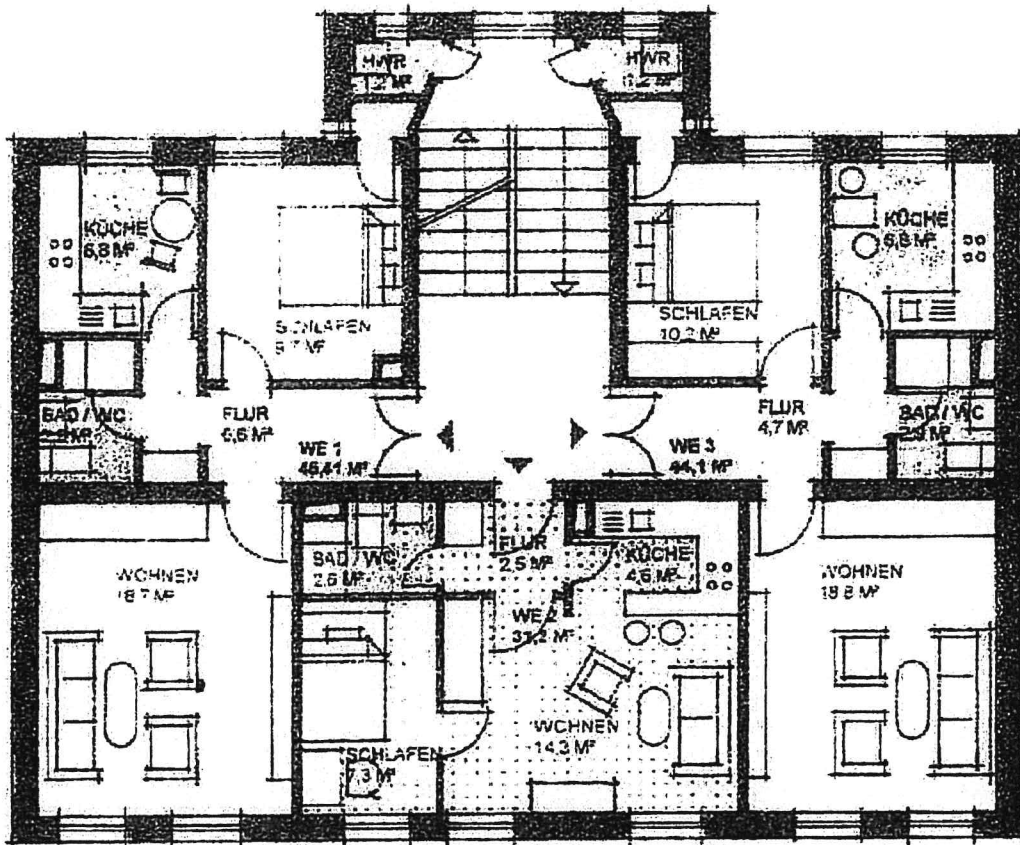
Grundriss 1 OG
