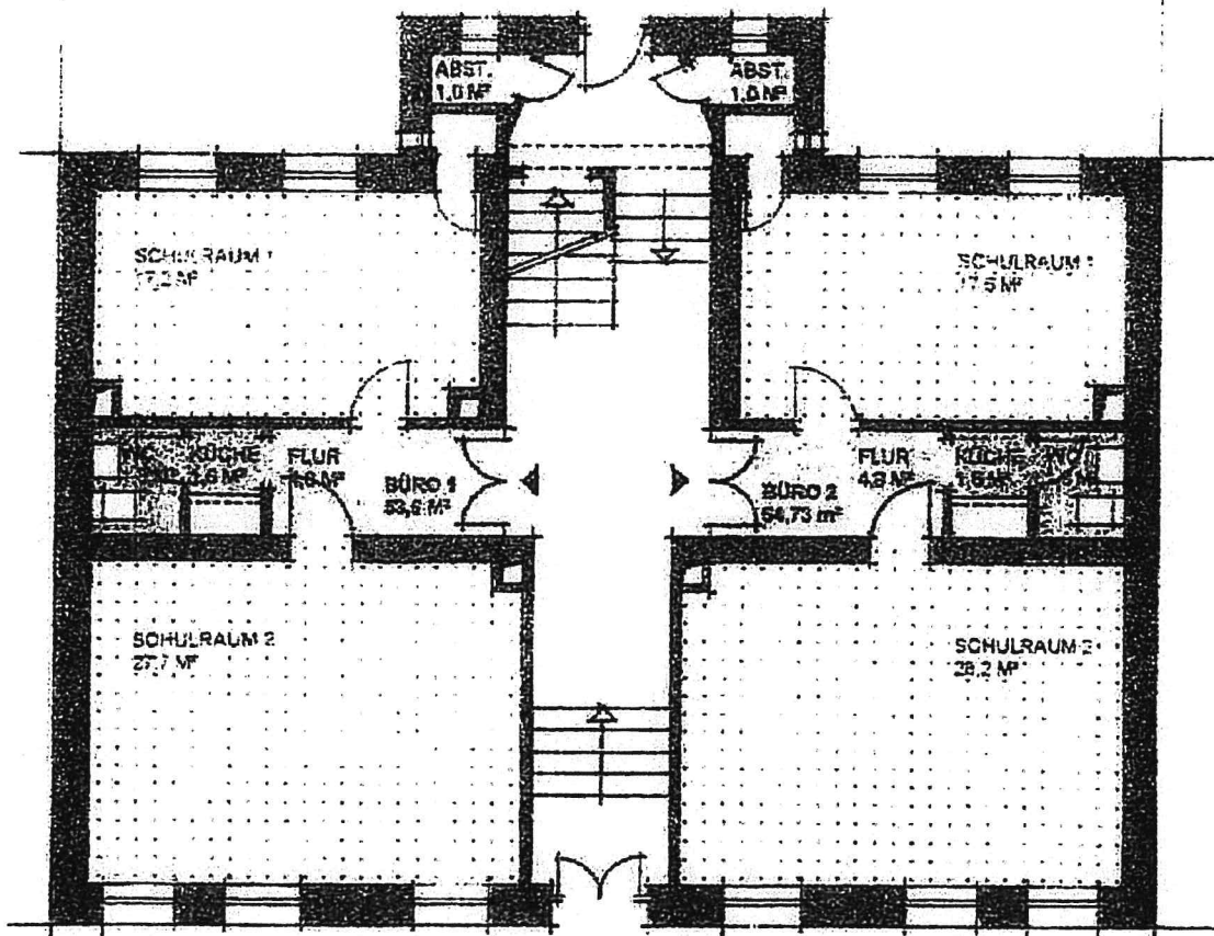
Grundriss EG m 1 100
