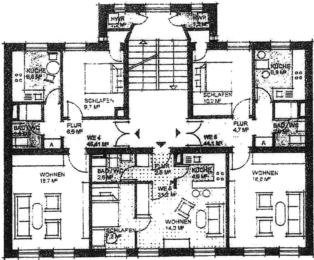
Grundriss 2.OG
