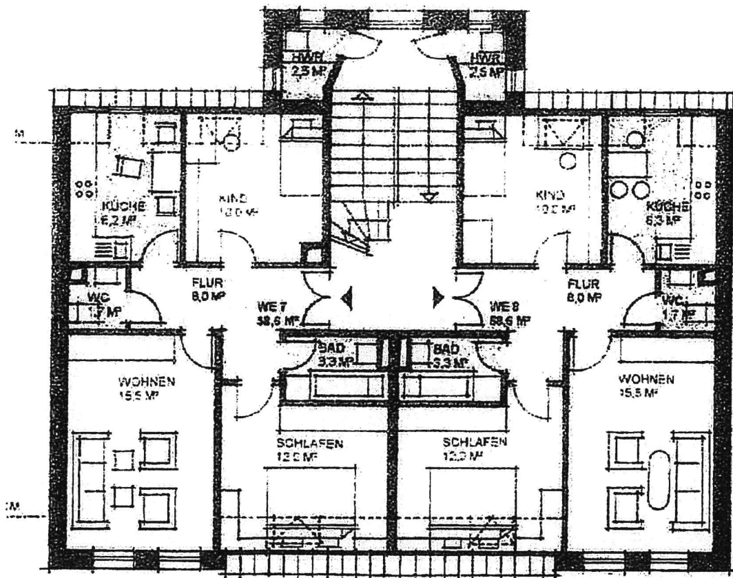
Grundriss DG
