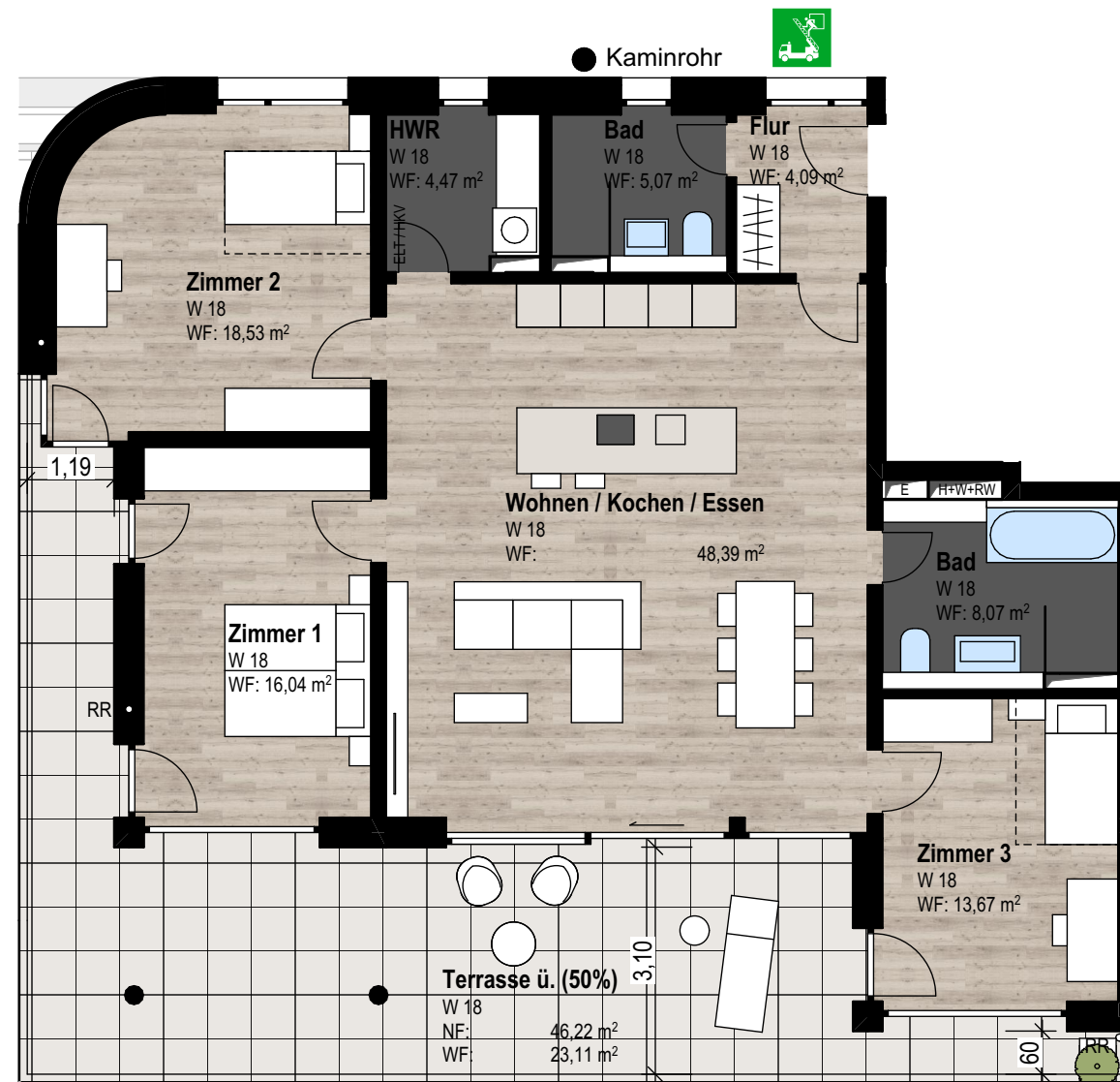
W 18 M1:100
