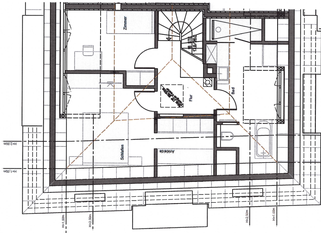
2. Dachgeschoss
