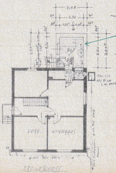
ERDGESCHOSS
