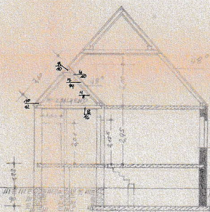
SCHNITT
