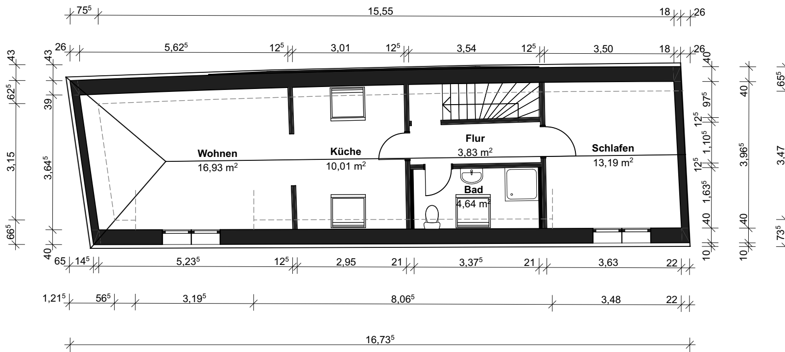
Dachgeschoß
