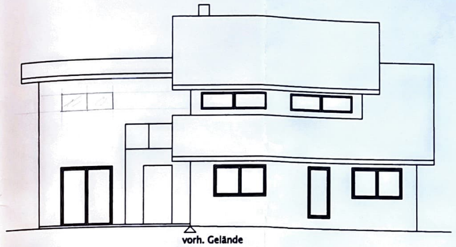
Ansicht Ost M.1:100
