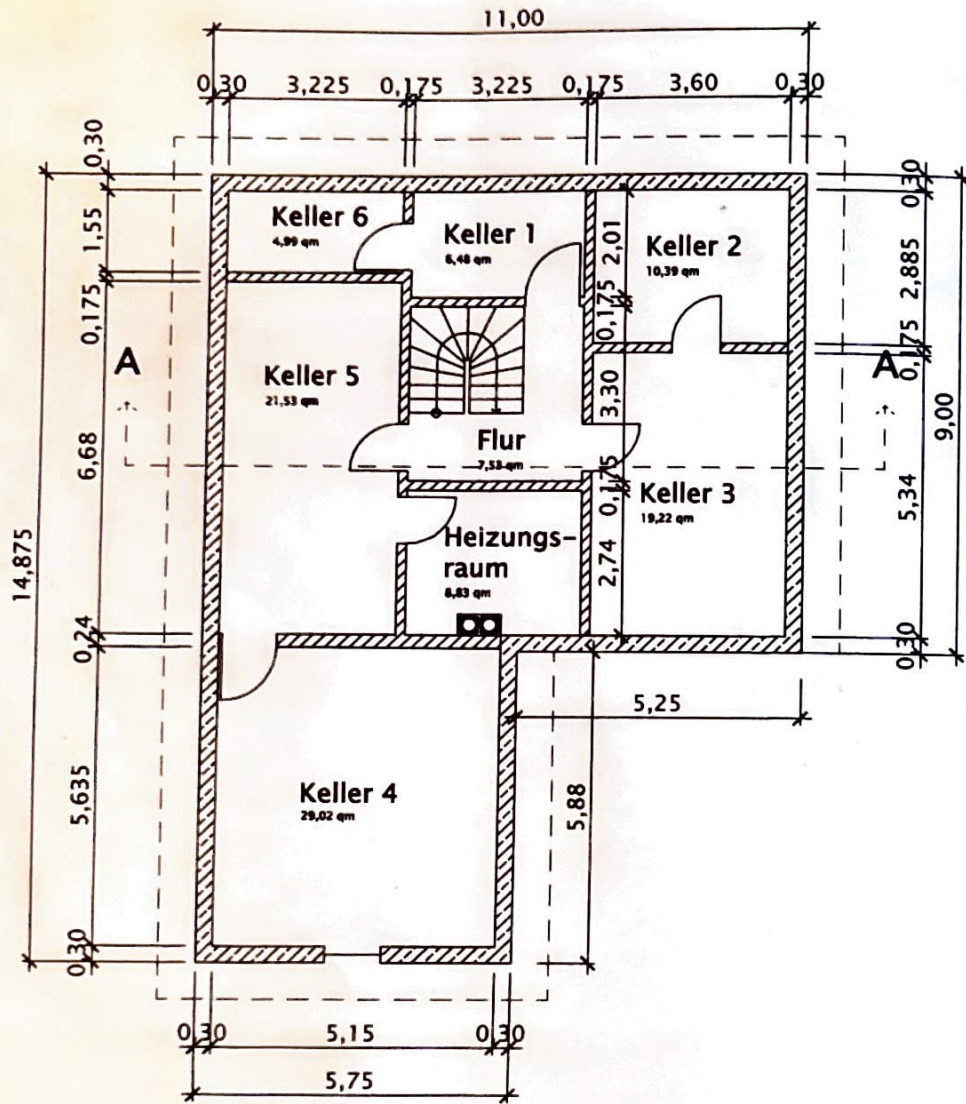
Kellergeschoß M.1:100
