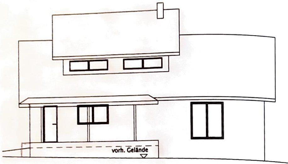
Ansicht West M.1:100
