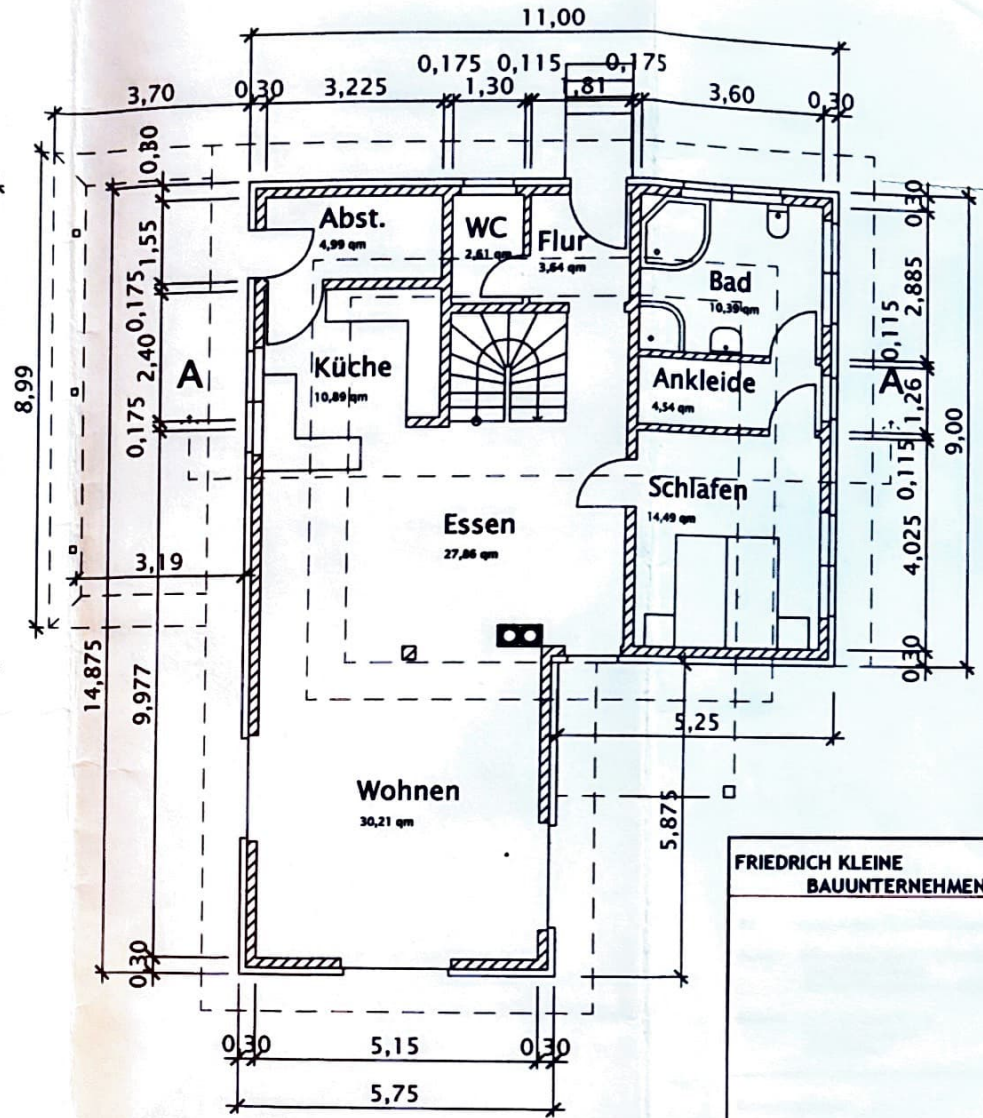
Erdgeschoß M.1:100
