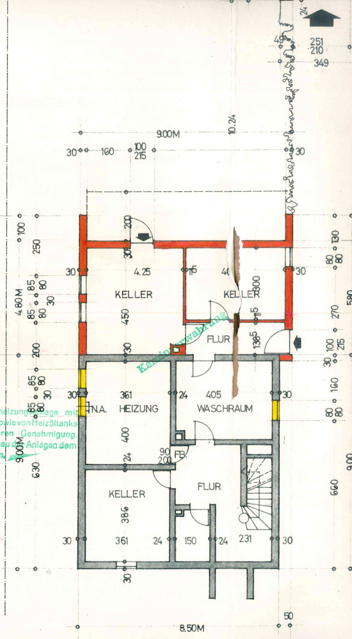
KELLERGESCHOSS
