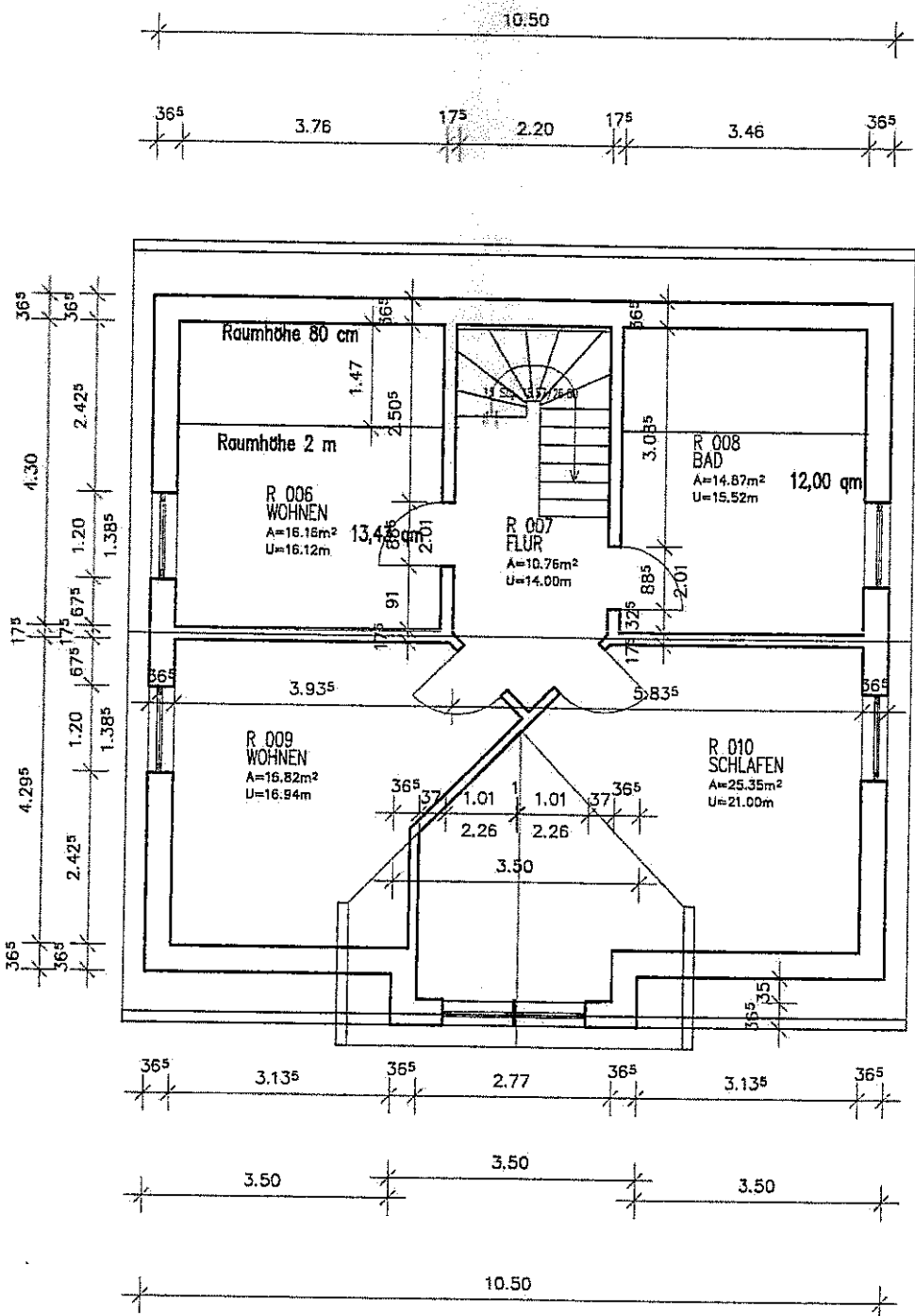
GRUNDRISS DG
