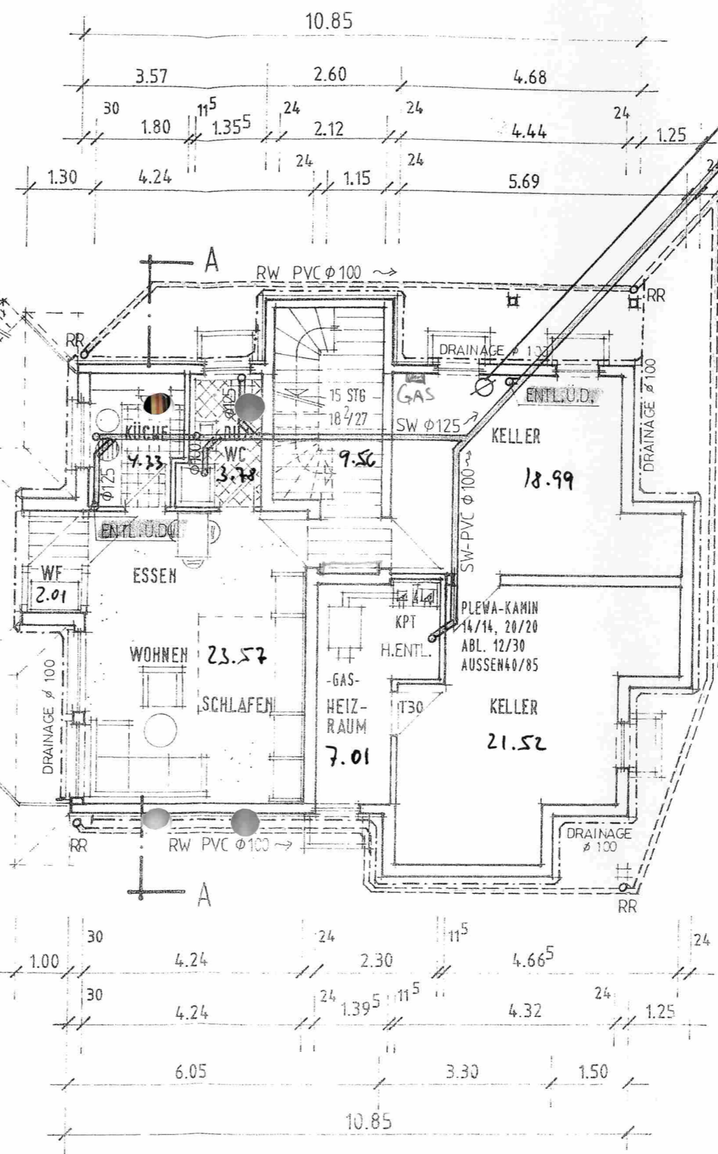
UNTERGESCHOSS M. 1 : 100
