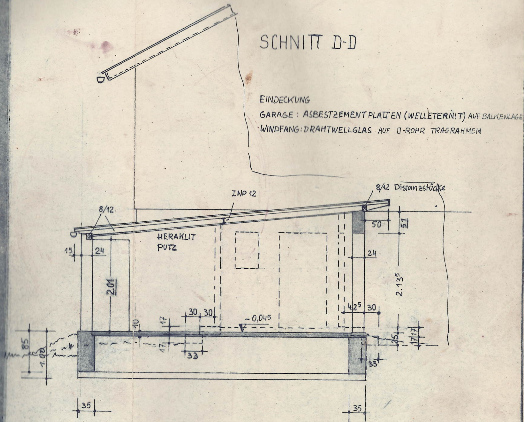
SCHNITTE, M 1:50
