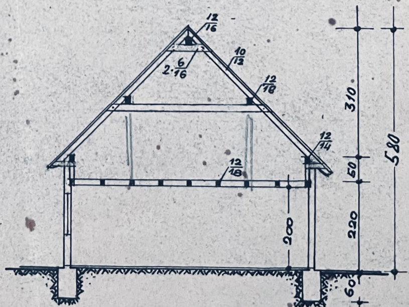
SCHNITT
