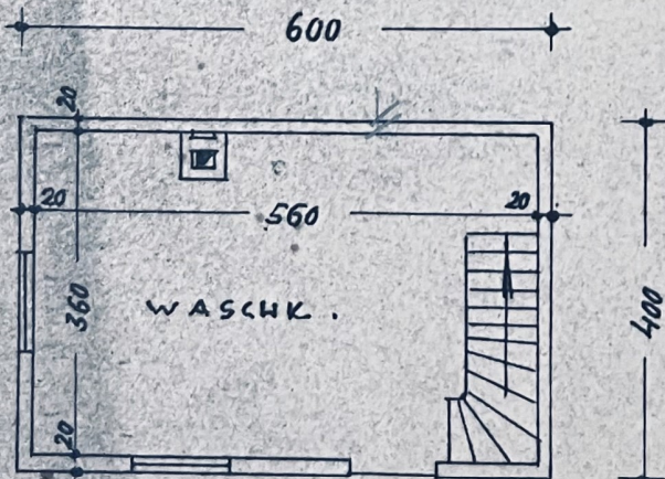
GRUNDRISS
