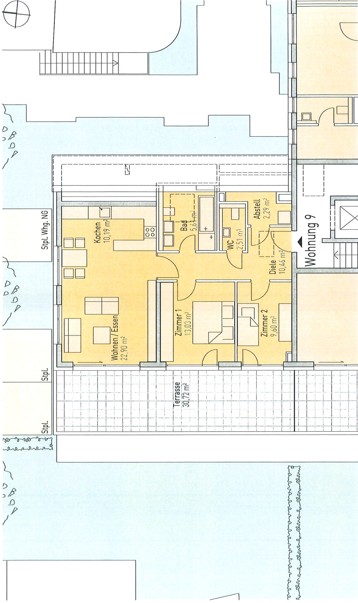
Wohnung Nr. 9 3-Zimmer-Wohnung Dachgeschoss
