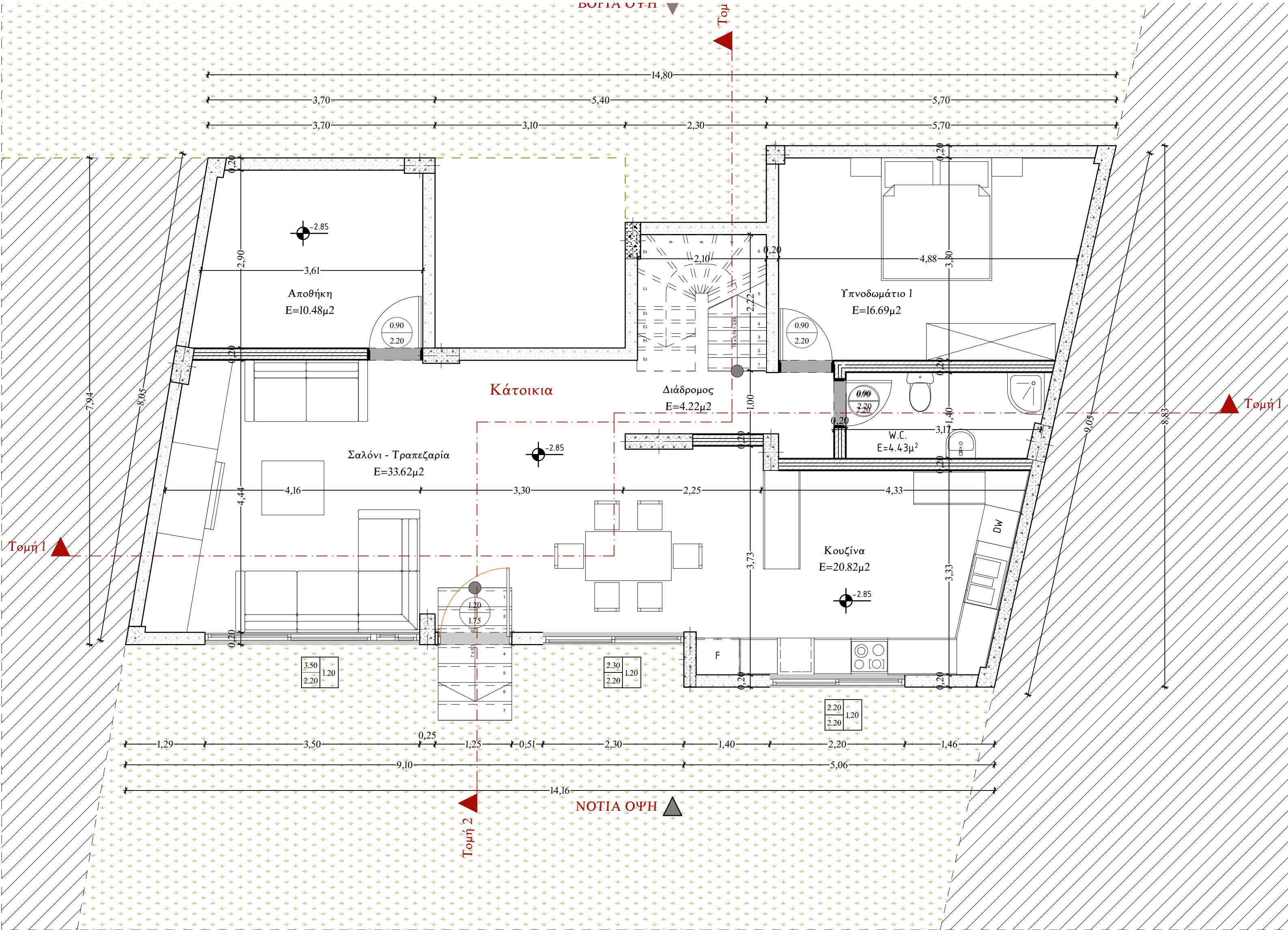
1 Κάτοψη Υπογείου 1:50
