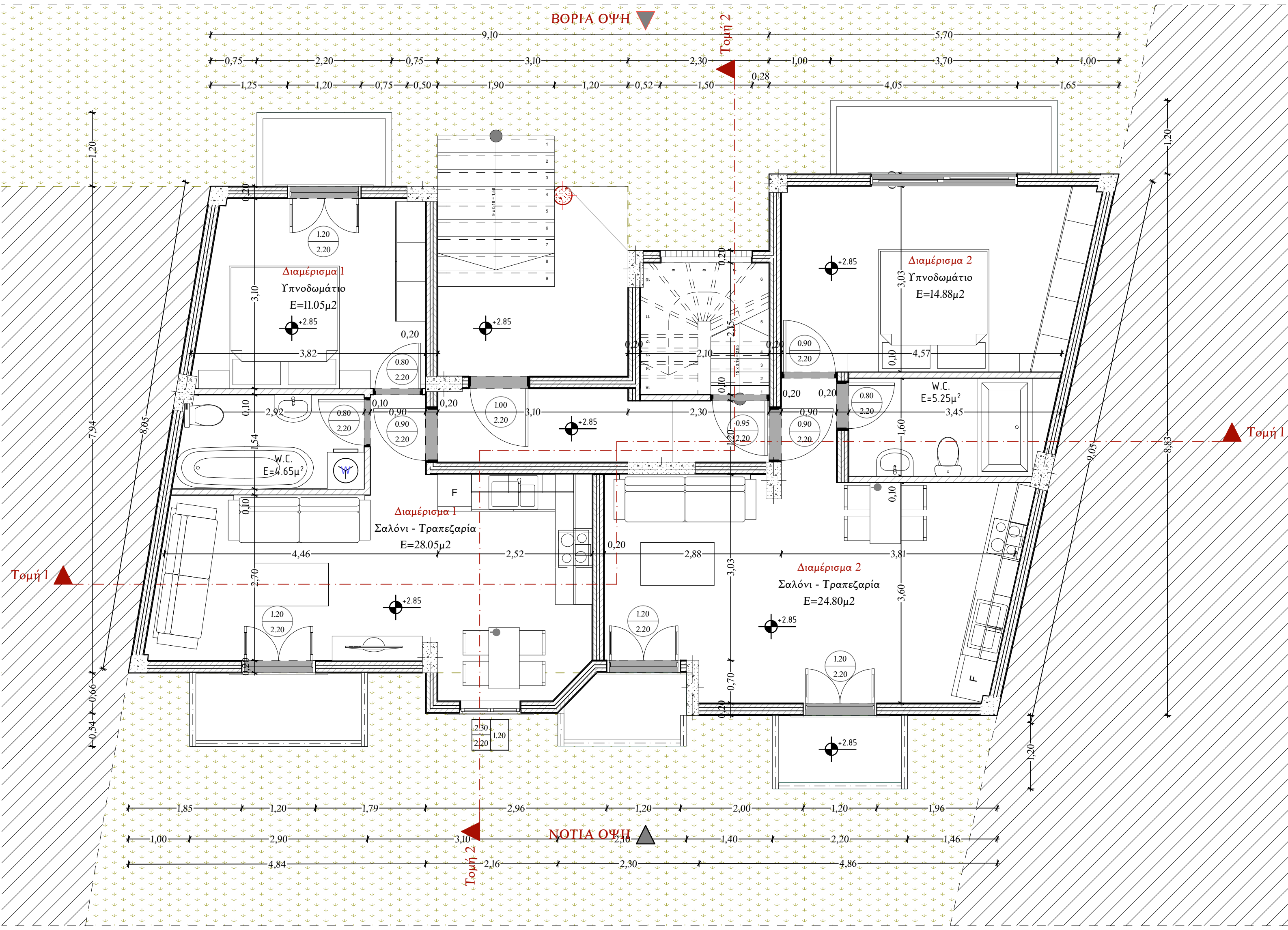
3 Κάτοψη Α Ορόφου 1:50
