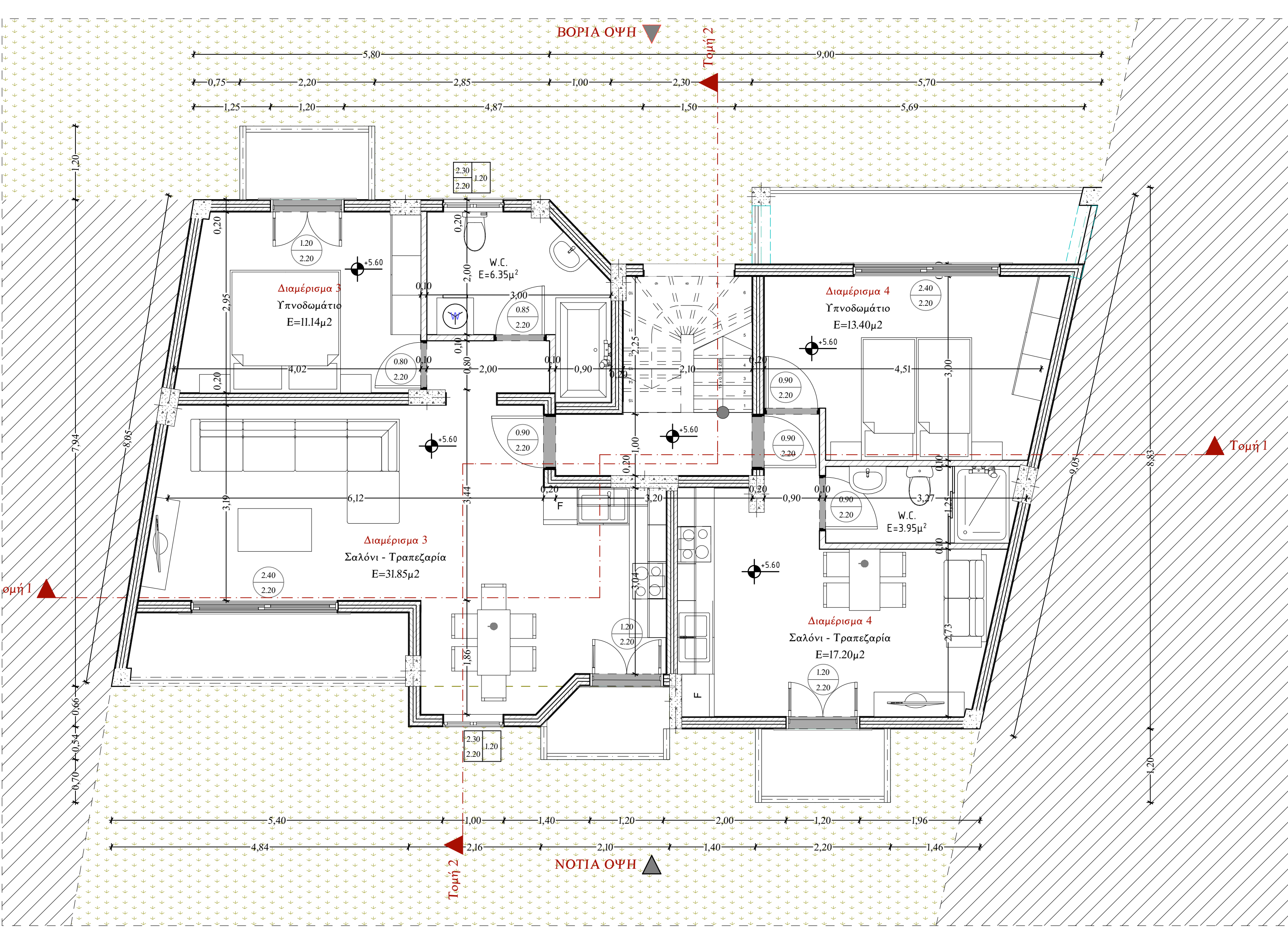
4 Κάτοψη Β Ορόφου 1:50
