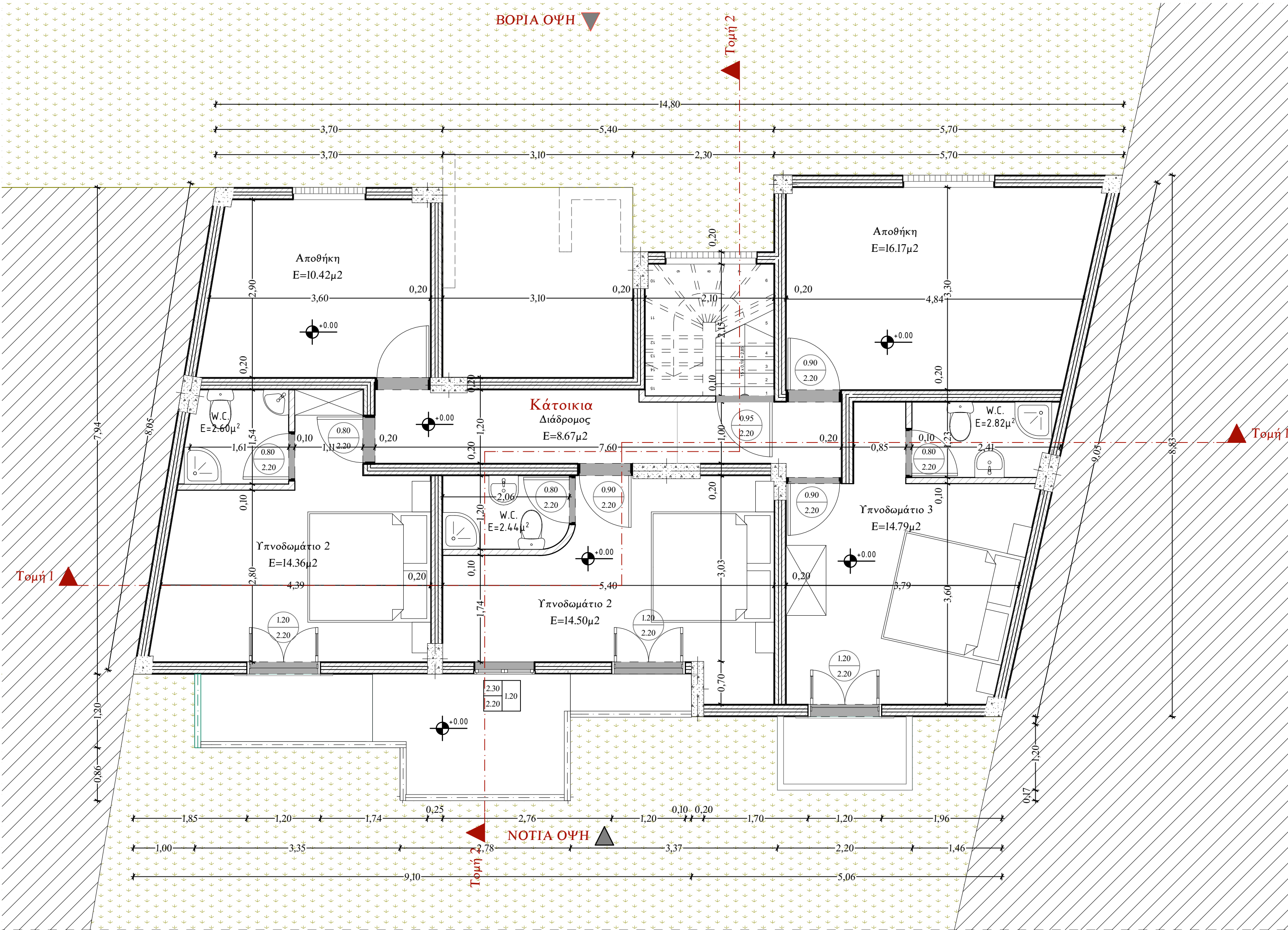
2 Κάτοψη Ισογείου 1:50
