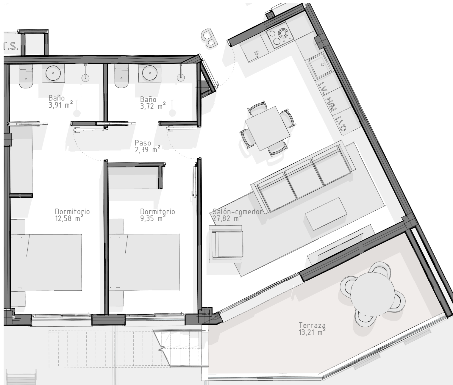
Esc.1. Viv B. Planta 2ª
