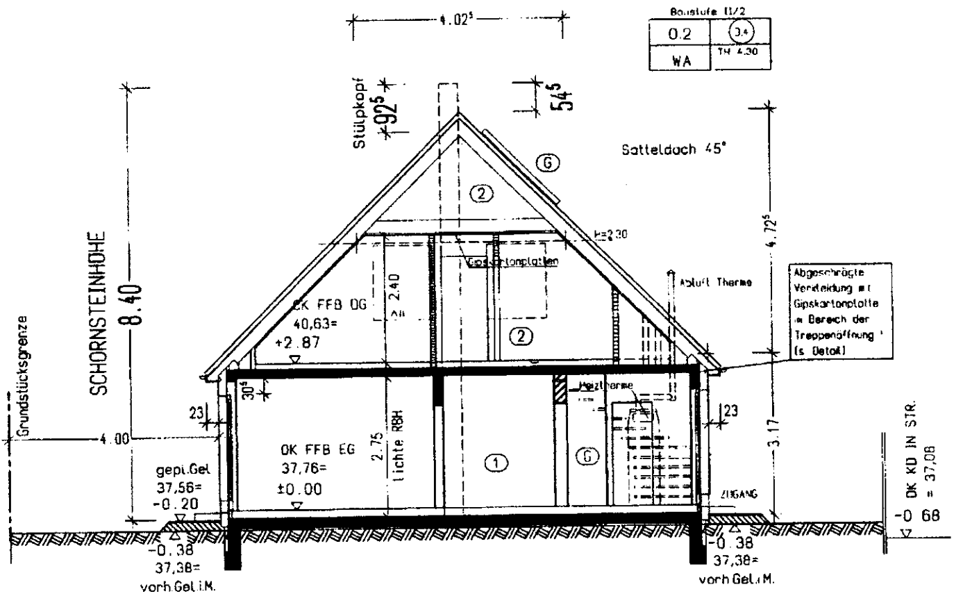
SCHNITT A-A
