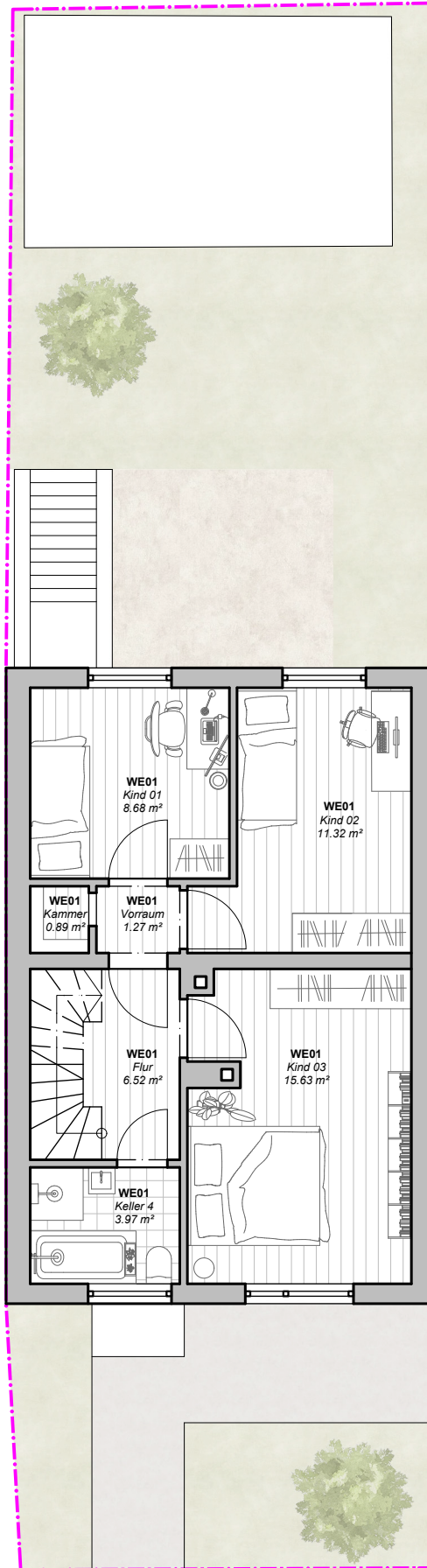
Grundriss 1. Obergeschoss
