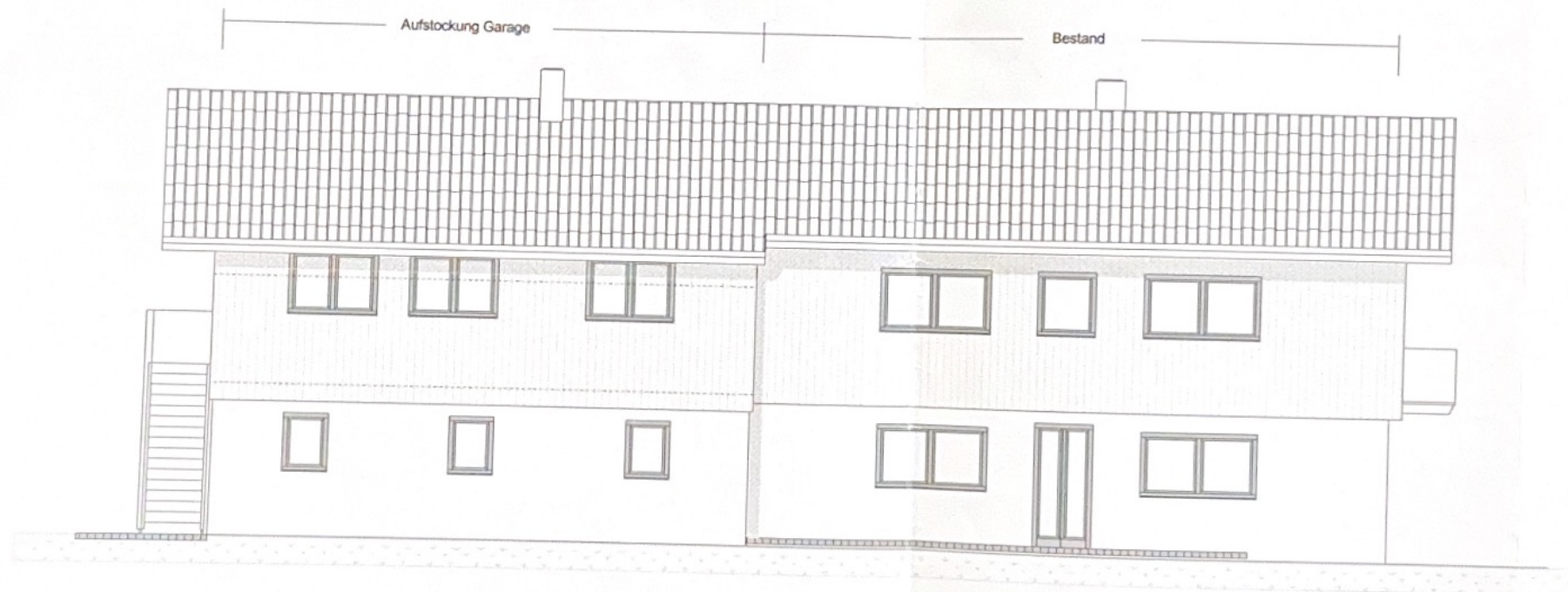
Ansicht Süd
