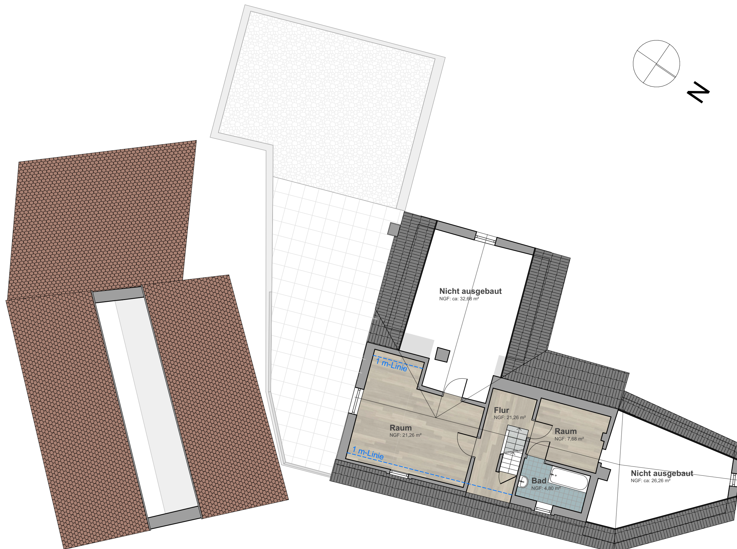
Grundriss DG
