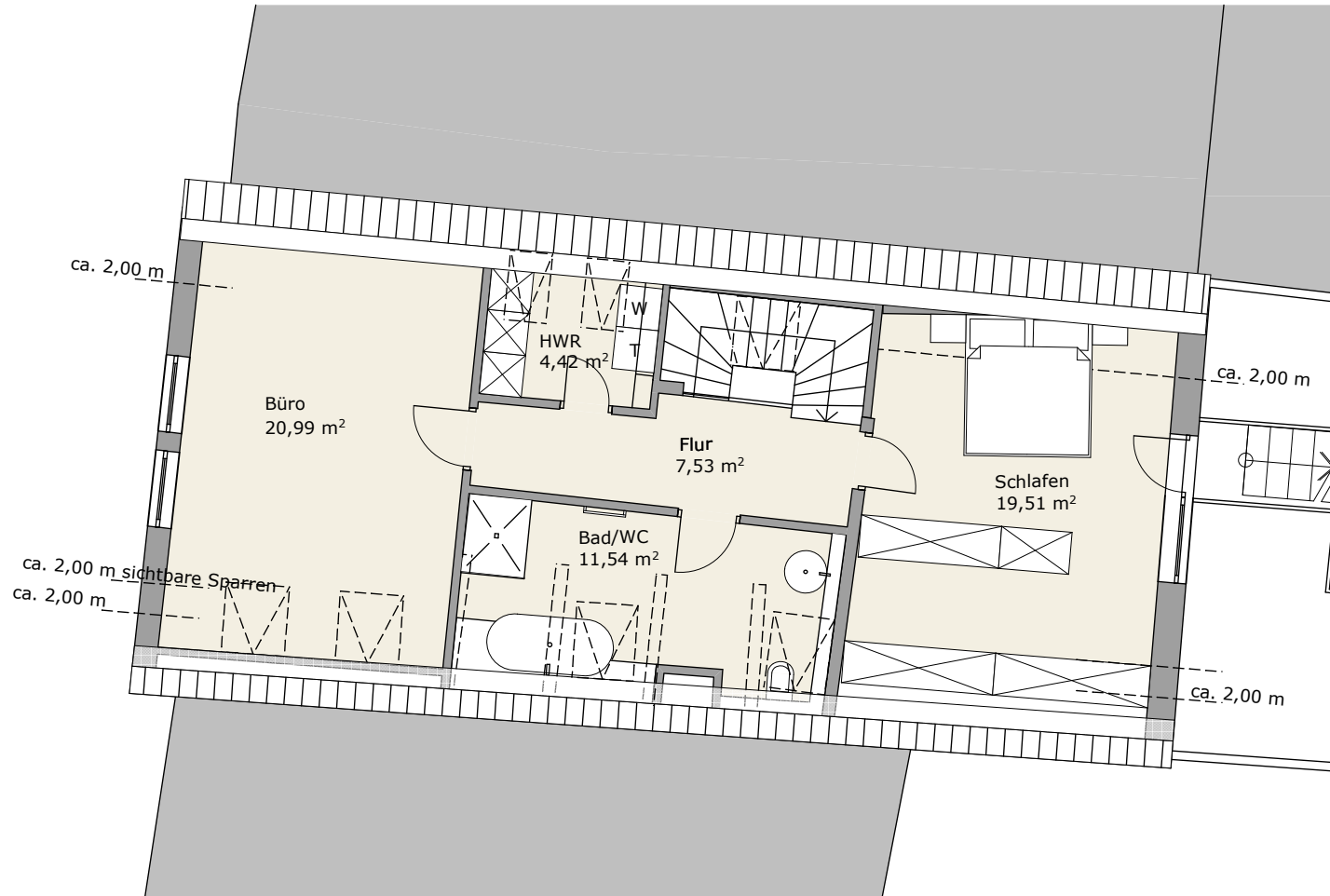
Dachgeschoss Variante 1
