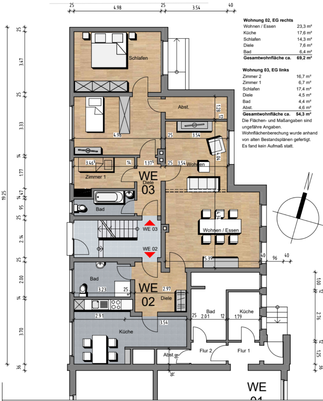
Grundriss Wohnungen 02 & 03
