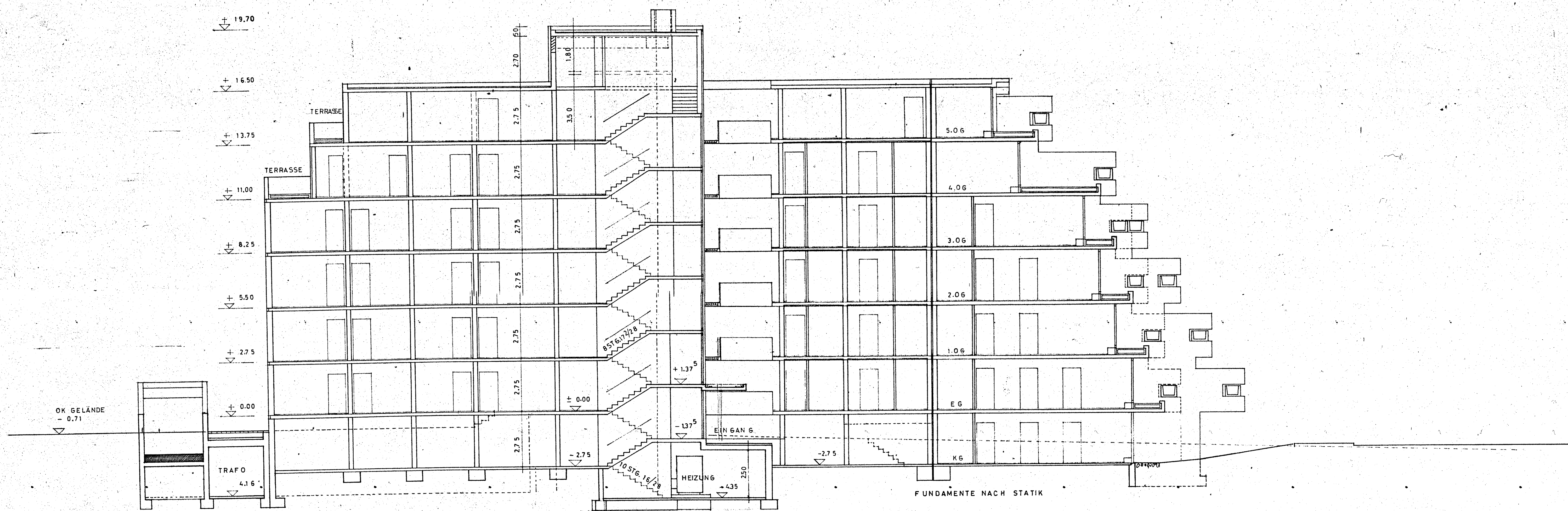
SCHNITT A-A
