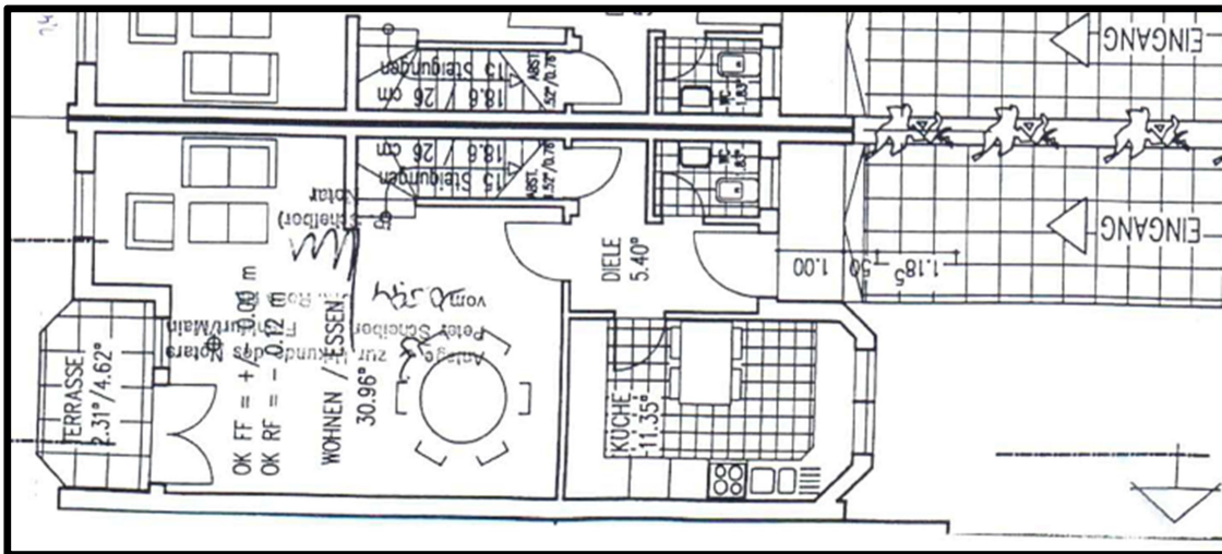
Erdgeschoss
