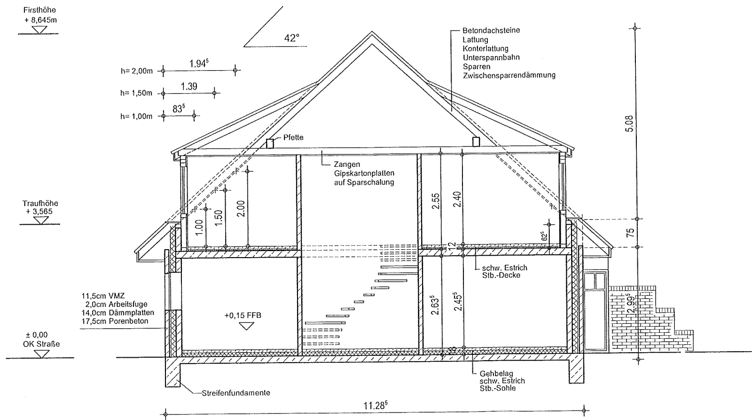
SCHNITT I-I
